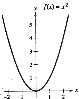
Quadratic Function
