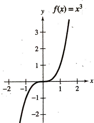
Cubic Function
